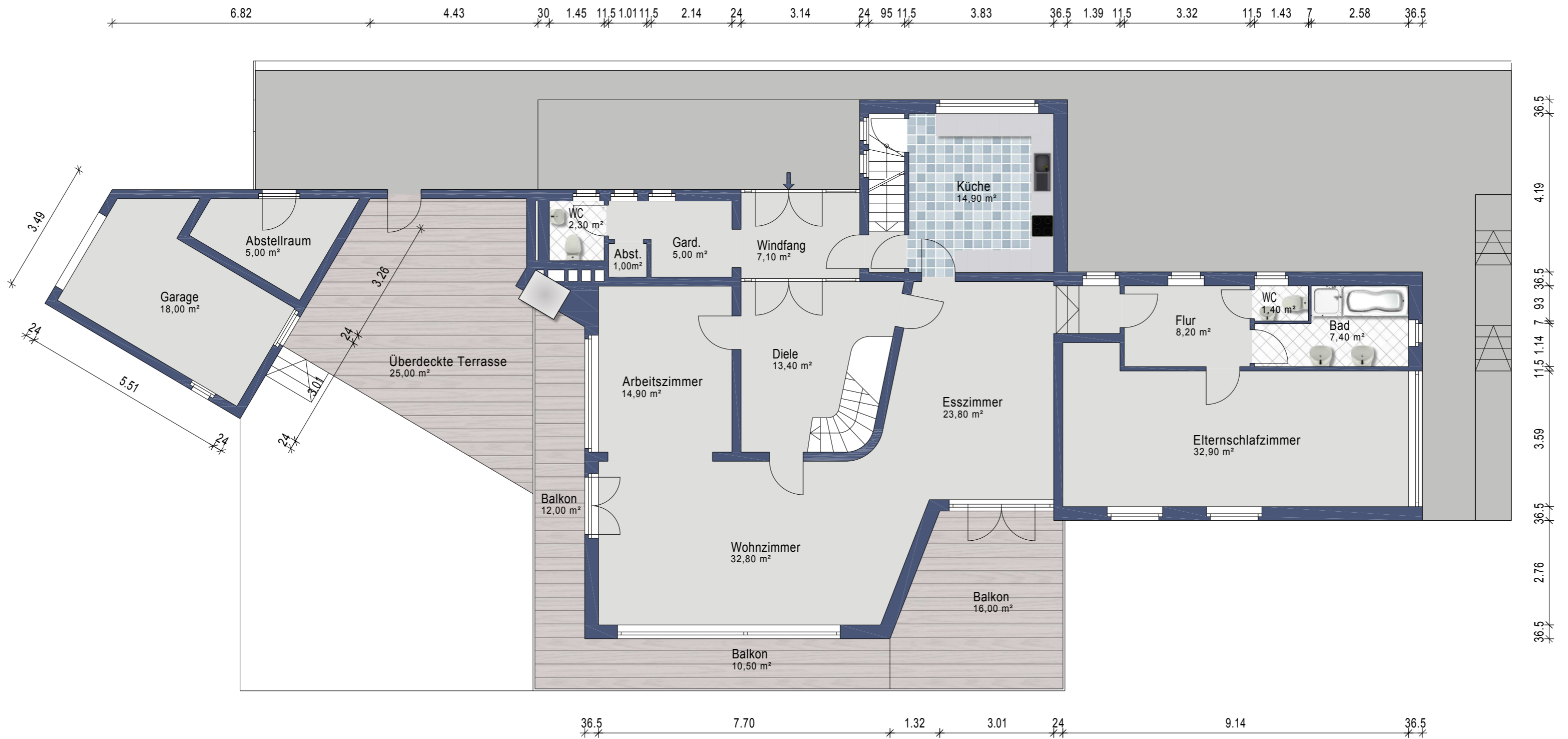
Erdgeschoss
